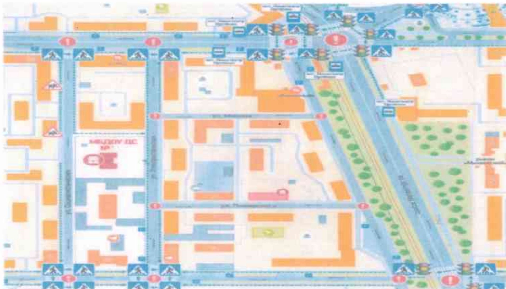
Схема № 2. Организация дорожного движения в непосредственной близости от МБДОУ «ДС № 206 г. Челябинска» СП 1 с размещением соответствующих технических средств организации дорожного движения, маршруты движения детей и расположение парковочных мест.
